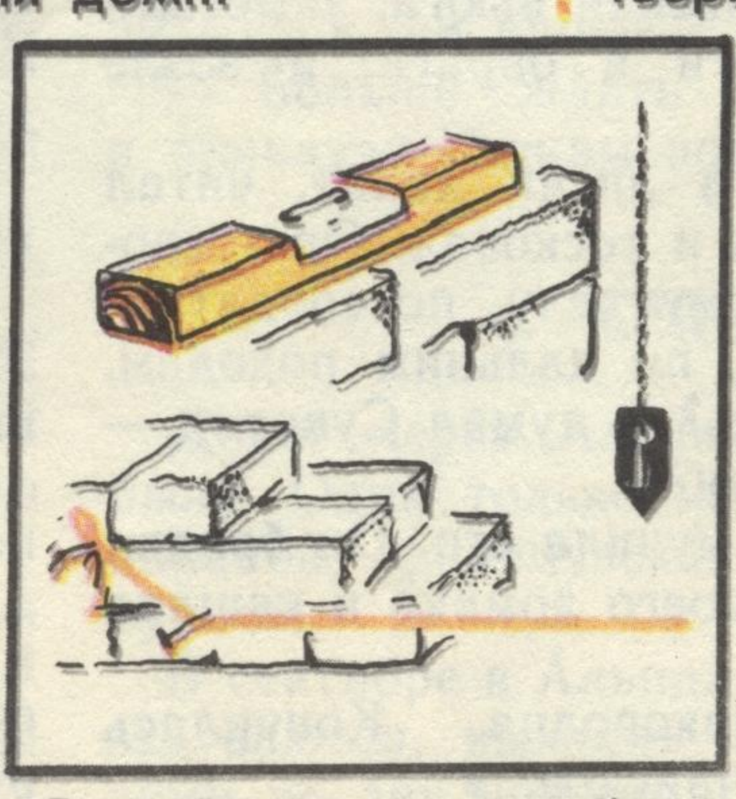
Проверяйте качество кладки 1) шнуром-причалкой, 2) отвесом, 3) используя деревянный уровень.
